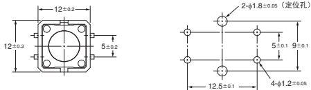
端子配置/内部连接图 （TOP VIEW）
