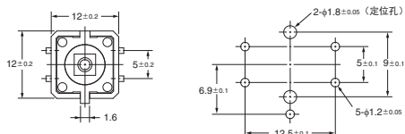
端子配置/内部连接图 （TOP VIEW）
